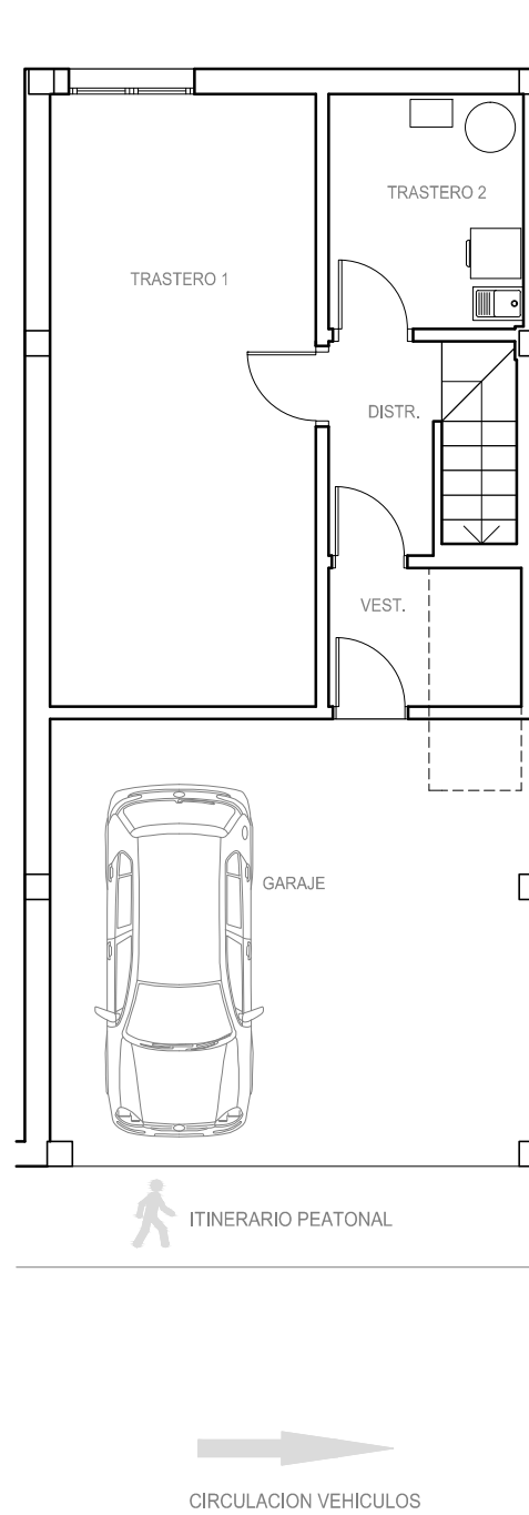
PLANTA SOTANO
