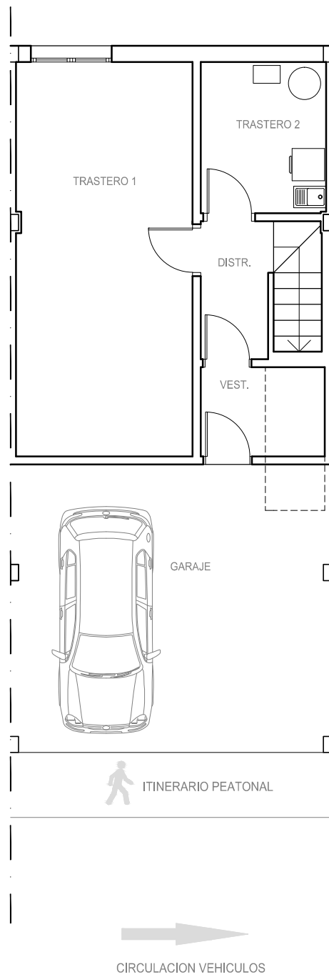
PLANTA SOTANO
