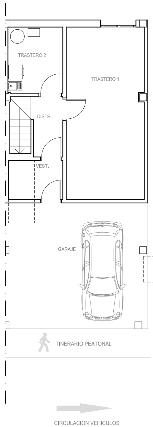
PLANTA SOTANO
