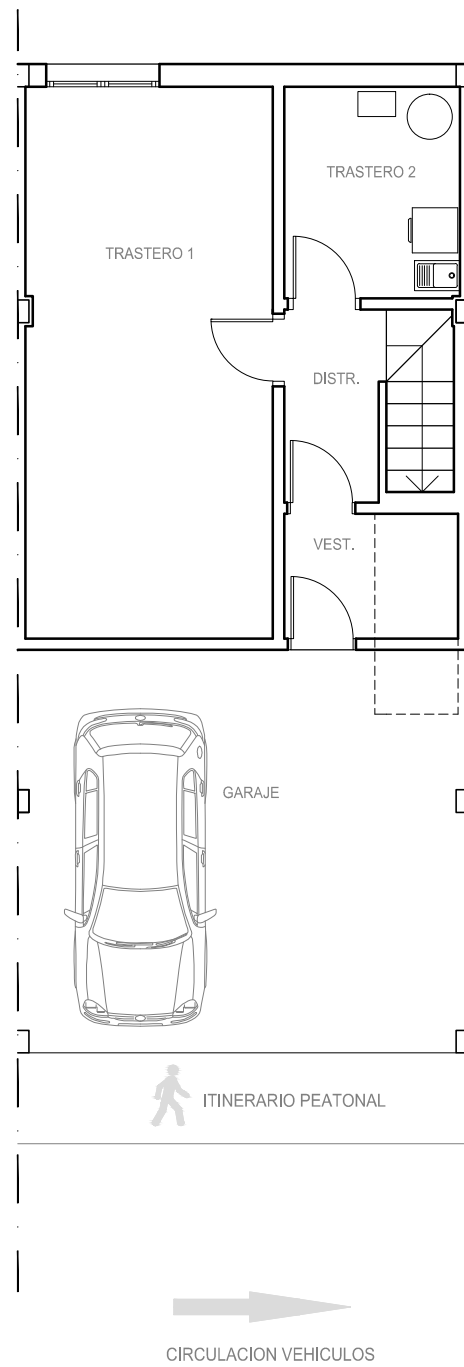
PLANTA SOTANO
